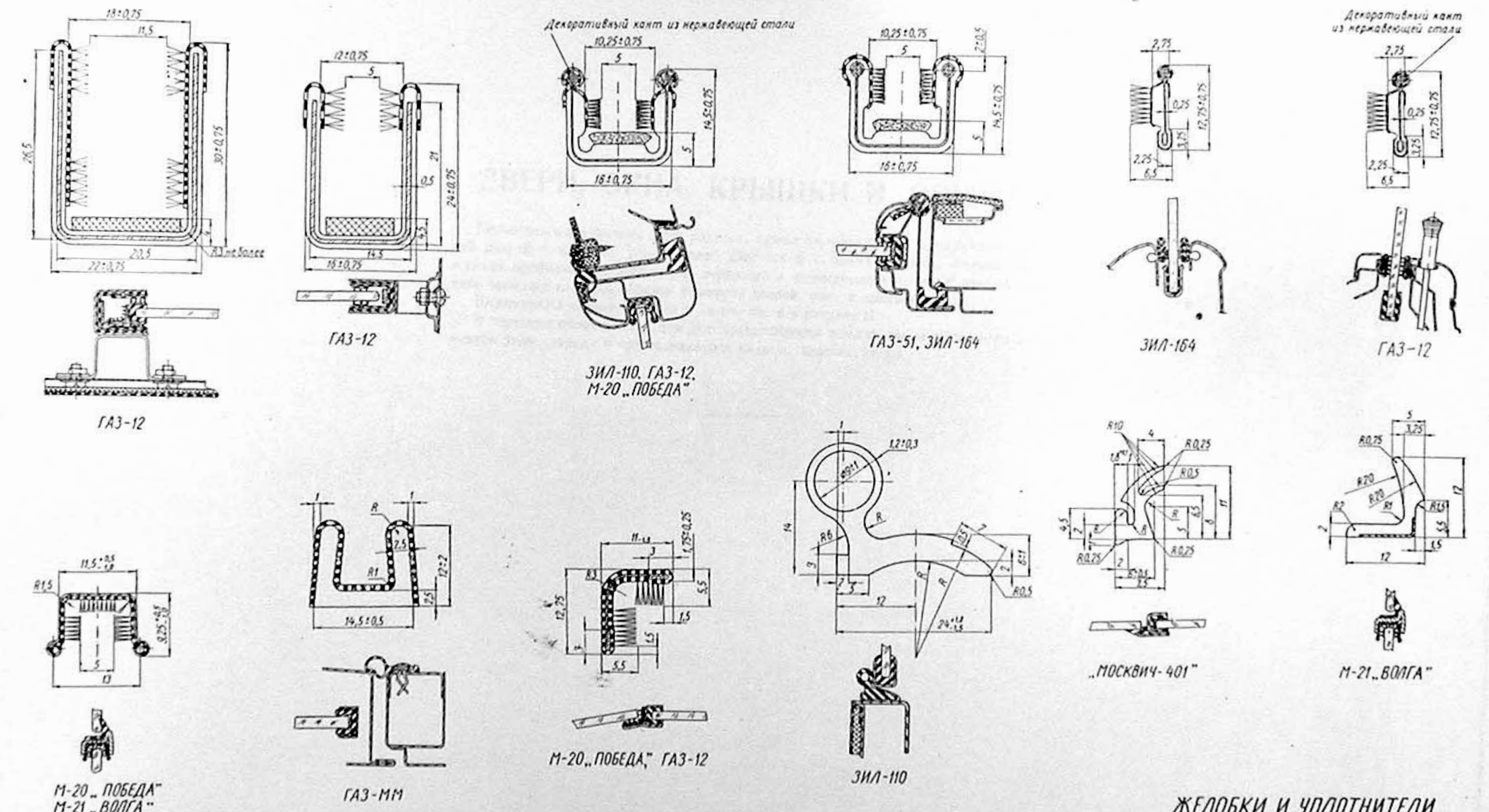
ЖЕЛОБКИ И УПЛОТНИТЕЛИ ДЛЯ ОТКРЫВАЮЩИХСЯ ОКОН
